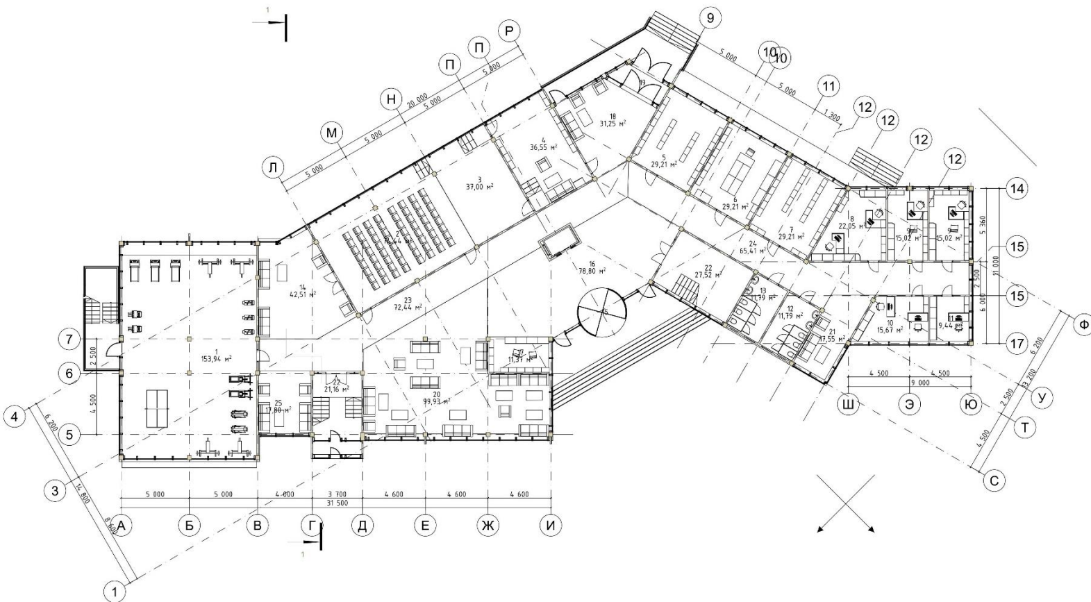
План Приміщень 1го поверху М 1:200
