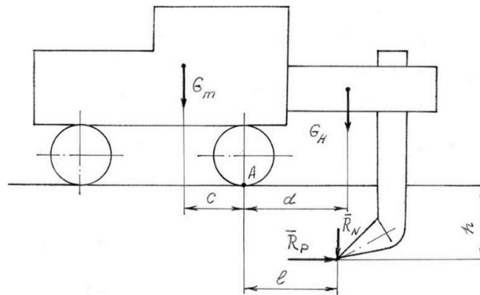
Рис. 1. Розрахункова схема розпушувального обладнання
