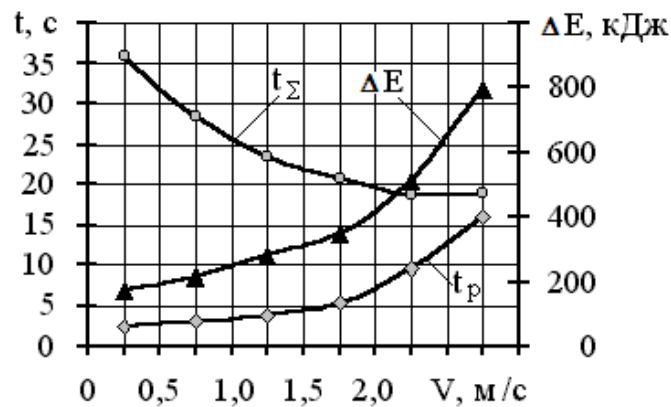
Рис. 2. Графіки зміни \Delta E , t_p і t_{\Sigma} від номінальної швидкості крана V
