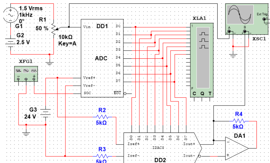
Рис. 1. Дослідження подвійного перетворення АЦП-ЦАП
