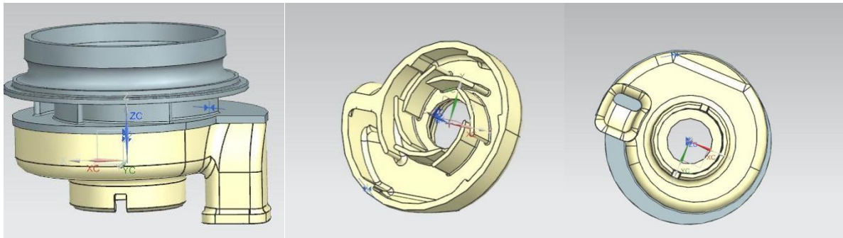
Рис. 2. 3D-модель завихрителю для потреб камери згорання двигуна літаку
