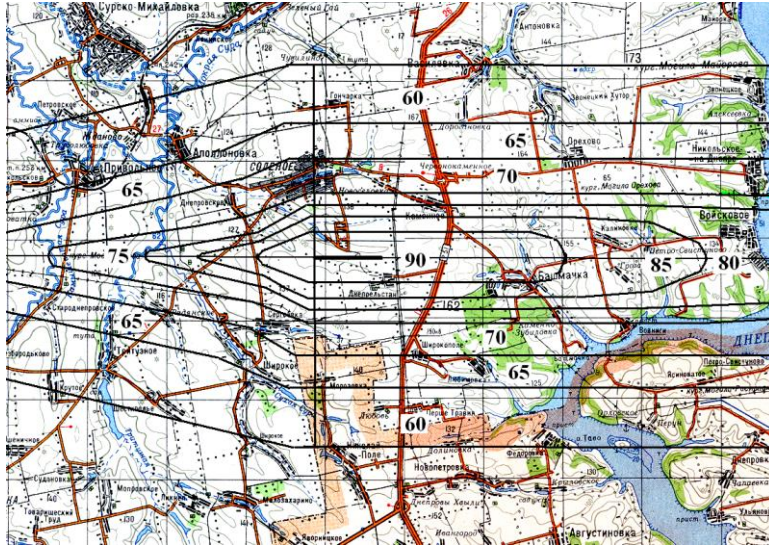
Рис. 2. Фрагмент карти шумового забруднення території навколо аеропорту.
