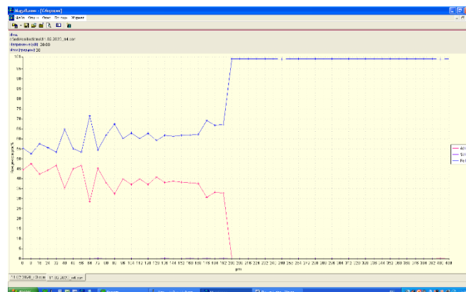
Рис. 2. Ренгенограмм алюмінідного покриття: (нижня лінія-алюміній, верхня лінія-залізо)
