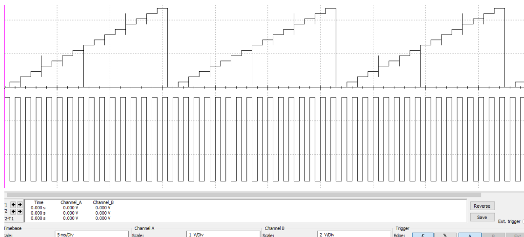
Рис. 2. Осцилограми роботи схеми ЦАП на основі лічильника і матриці R-2R
