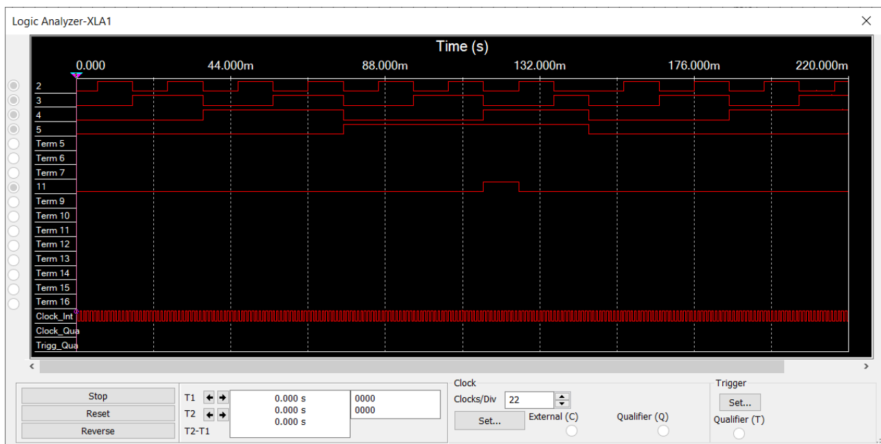
Рис.2. Часові діаграми роботи пристрою
