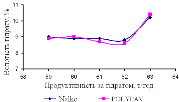
Рис. 3. Порівняння впливу зневоднювачів Nalko 85488 і POLYPAV-C16 на вологість гідроксиду алюмінію при різній продуктивності за гідратом
