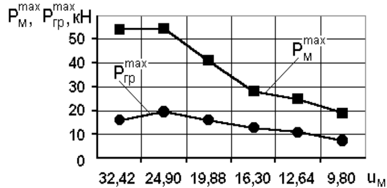
Рис. 1. Графіки зміни навантажень P_M^{\max} і P_{гр}^{\max} від передаточного числа u_M
