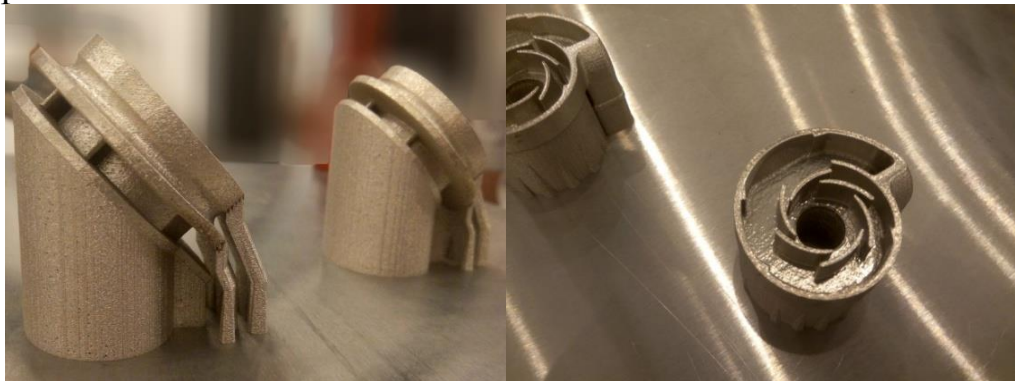
Рис. 3. Завихритель для потреб камери згорання двигуна літаку, вирощений за допомогою технології SLS зі сплаву Inconel 718
