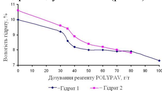
Рис. 2. Впливу дозування зневоднювача POLYPAV-C16 на вологість гідроксиду алюмінію при різних за складом гідратах
