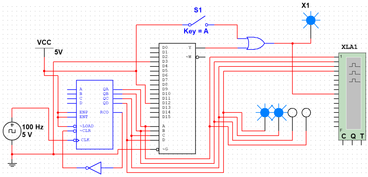
Рис.1. Схема пристрою в програмі Multisim 12
