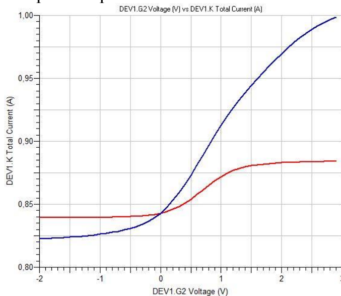
Рис. 2. Порівняння передавальних характеристик двозаслонного і однозаслонного комбінованих транзисторів
