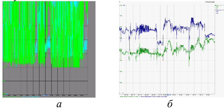
Рис.1. Реєстрація щільності шламу за показаннями щільноміра (а) і витрати флокулянта НХ-3000 та розбавленої пульпи (б) на згущувач
