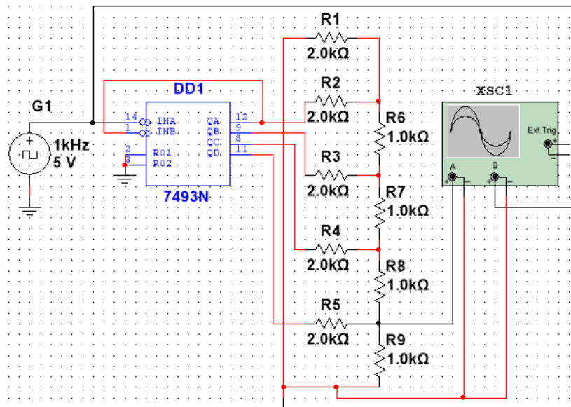
Рис. 1. Схема ЦАП на основі лічильника і матриці R-2R
