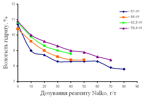
Рис. 1. Вплив дозування зневоднювача Nalko 85488 на вологість гідроксиду алюмінію за різної продуктивності фільтра за гідратом
