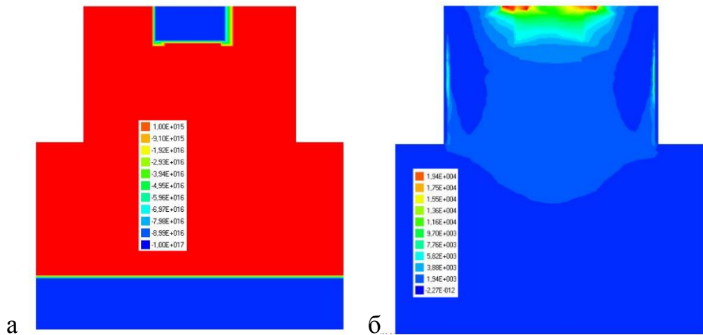
Рис. 1. Розподіл концентрацій легуючих домішок (а) і струму (б) у двозаслонном транзисторі
