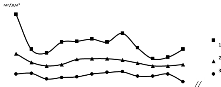
Рис. 2. Динаміка зміни значень вмісту сульфатних іонів води річки Случ. Цифрами на графіку показано: 1 – максимальне значення; 2 – середнє значення; 3 – мінімальне значення;
