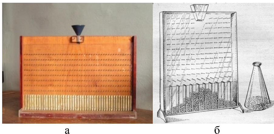
Рис. 1. Загальний вид дошки Гальтона (а) та статистична закономірність розподілу молекул (б)
