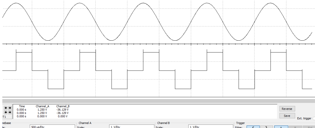
Рис.2. Осцилограми роботи схеми перетворення АЦП-ЦАП, F_d = 4 кГц
