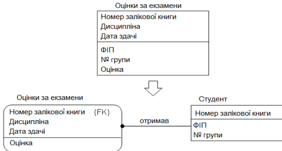
Рисунок 8.13 – Забезпечення повної функціональної залежності
