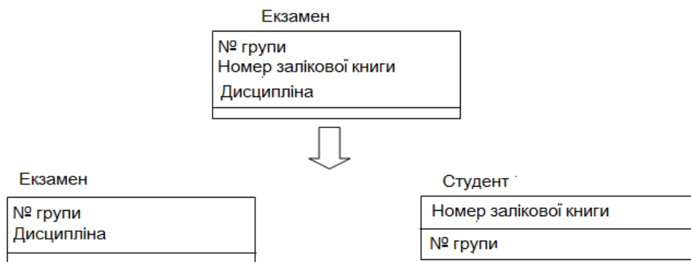
Рисунок 8.16 – Приведення відношення до 4NF
