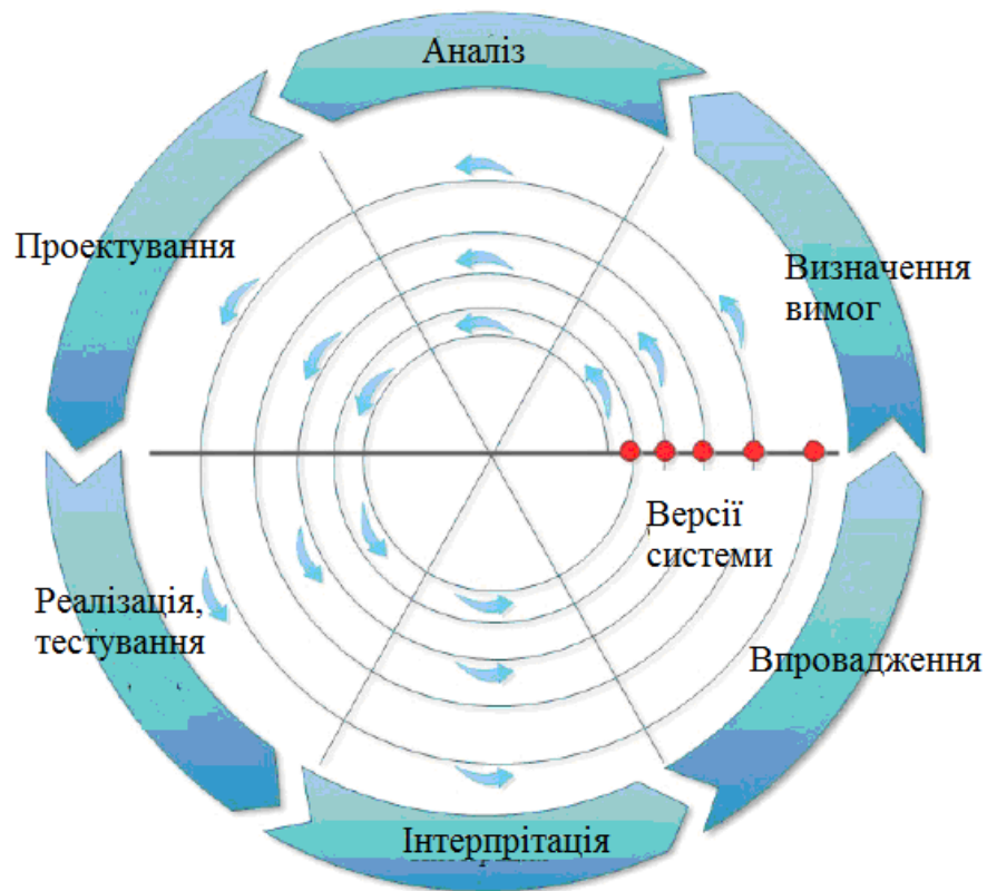
Рисунок 1.5 – Спіральна модель ЖЦ ІС
