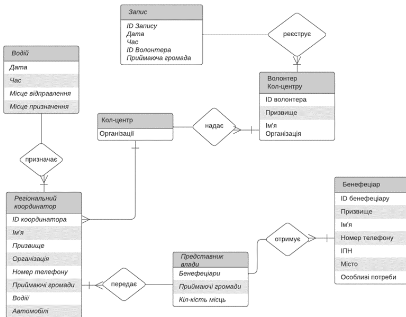
Рис. 2. ER-діаграма CRM система для евакуації цивільного населення
