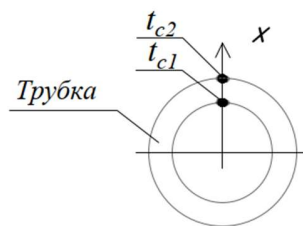
Рисунок 3.8- Лінійна зміна температура по товщині однорідної стінки
