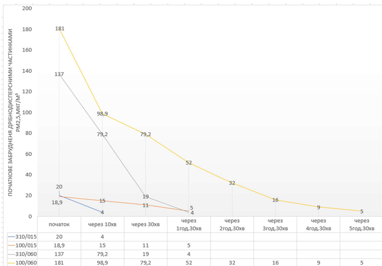
Рис.3.9. Показники очищення повітря в приміщенні при використанні рециркуляційного агрегату з змінною витратою повітря з фільтрувальною вкладкою типу HEPA11.
