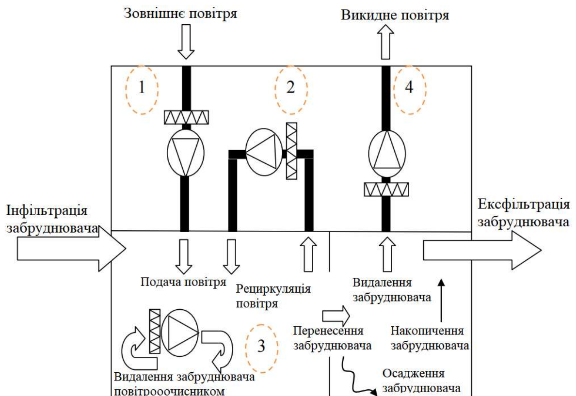
Рис.1.4. Схема видалення забруднювачів з будівлі за допомогою інженерних систем вентиляції та повітроочисників. На схемі вказано розміщення повітряних фільтрів на позиціях 1-4. Фільтр на позиції 1 – на припливній системі вентиляції, очищує зовнішнє повітря. Фільтр 2 – очищує рециркуляційне повітря, що циркулює через кондиціонер в приміщенні. Фільтр 3 – фільтри на повітроочиснику в приміщенні. Фільтр 4 – на витяжній системі вентиляції [27].
