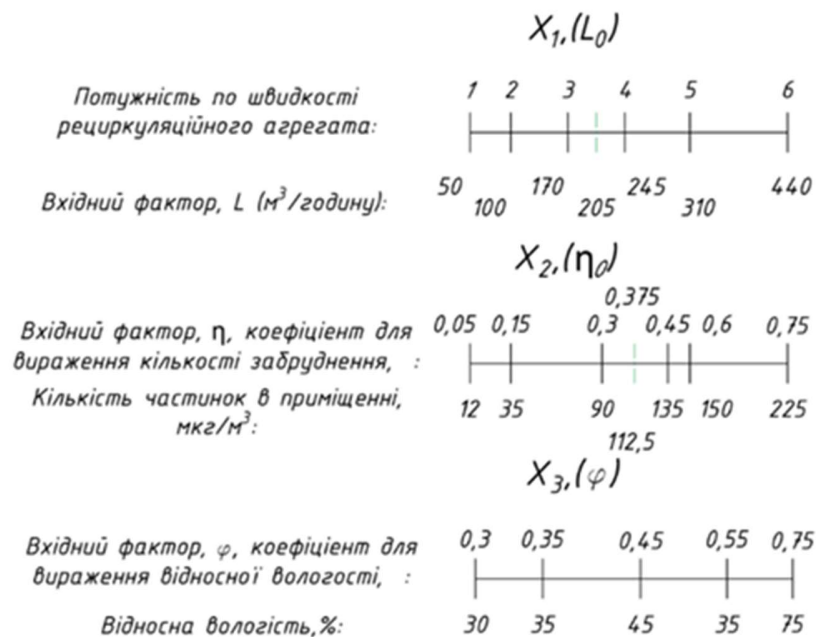
Рисунок 3.4. Центральні точки плану для ПФЕ при трьох факторах : X_1 -пропускна потужність повітрообробної установка ( 100 та 310 м 3 /год); X_2 -рівень початкового забруднення (15% та 60%); X_3 -відносна вологість (35% та 55%).
