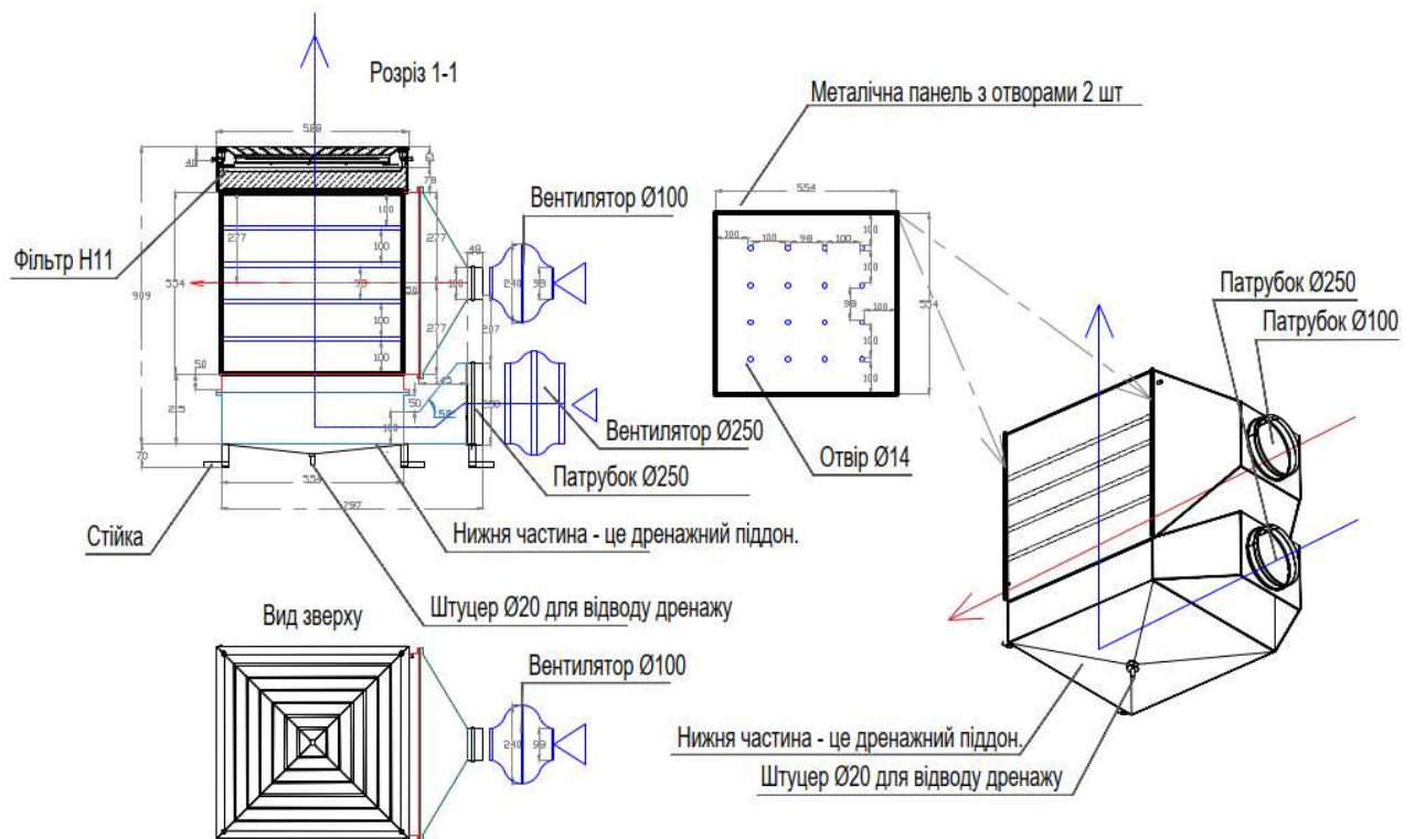
Рис 2.4. Модель очищувача повітря рециркуляційного типу з вставкою HEPA 11 та теплообмінником «повітря-повітря».
