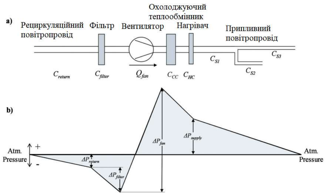
Рис.1.10. Розподіл тиску в системі ОВК: (а) схема системи, (б) розподіл статичного тиску [126].
