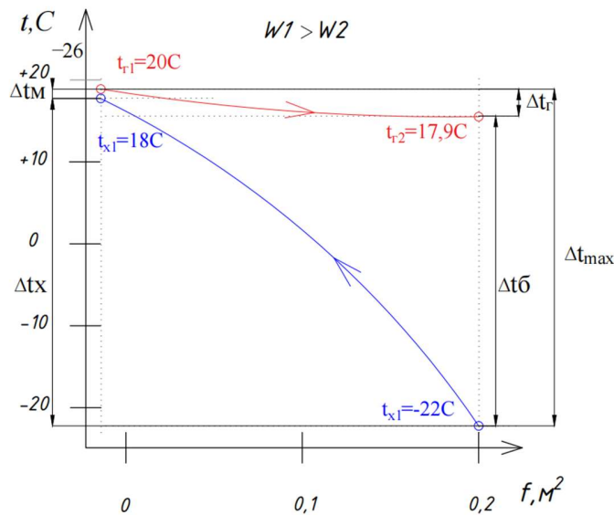
Рис 2.3 Зміна температур теплоносіїв на поверхні теплообмінника при протитечії. f , m^2 – площа теплообміну з боку гарячого та холодного теплоносія.
