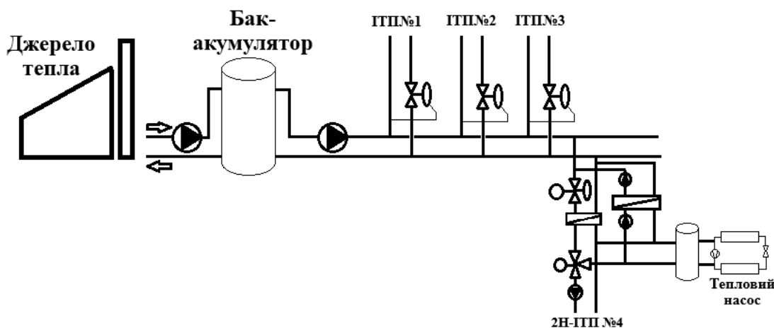
Рис.3.3 Структура системи внутрішнього тепlopостачання офісної будівлі Danfoss Україна
