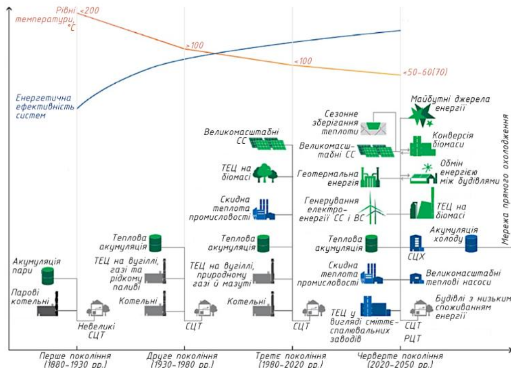
Рис.1.1 Еволюція систем ЦТ в чотирьох поколіннях з концептуальним графіком енергетичної ефективності та рівня температури залежно від часу, року: СЦТ або ЦТ – системи централізованого теплопостачання; СЦХ або ЦХ – системи централізованого холодопостачання; РЦТ – розроблення (покоління) централізованого теплопостачання та енергетичних систем/період найкращих доступних технологій.
