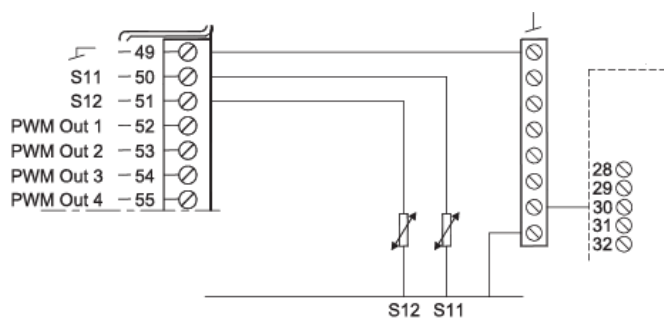
Рис.4.14 Схема підключення датчиків температури до модулю розширення
