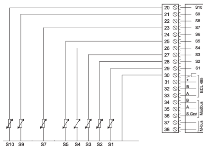
Рис.4.13 Схема підключення датчиків температури до клемної панелі
