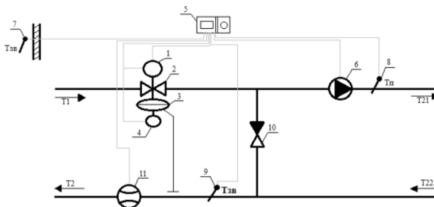
Рис.1.21 Принципова схема залежного приєднання ТП четвертого покоління.
