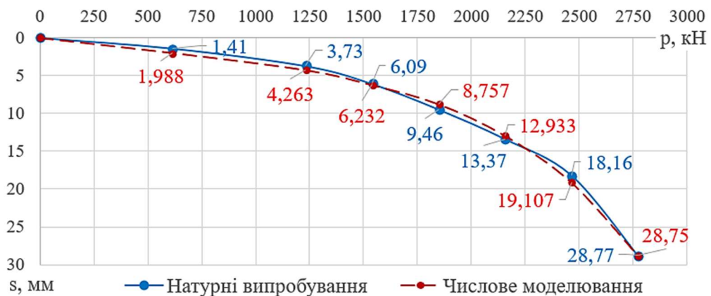
Рис. 3 Графік S = f(p) за даними натурних випробувань палі та результатами числового моделювання випробування
