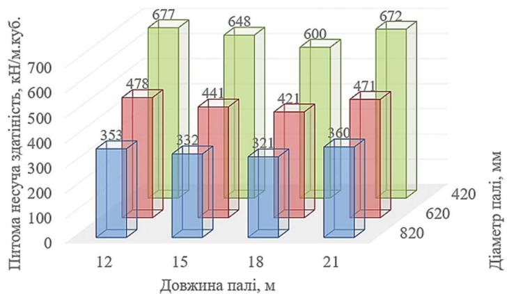
Рис. 6. Питома несуча здатність палей F''_d , кН/м³
