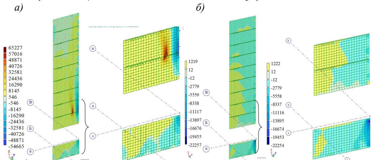
Рис. 10. Поздовжні зусилля N_y , \text{кН/м}^2 в стінах секції будинку: а – квазістатична постановка; б – динамічна постановка
