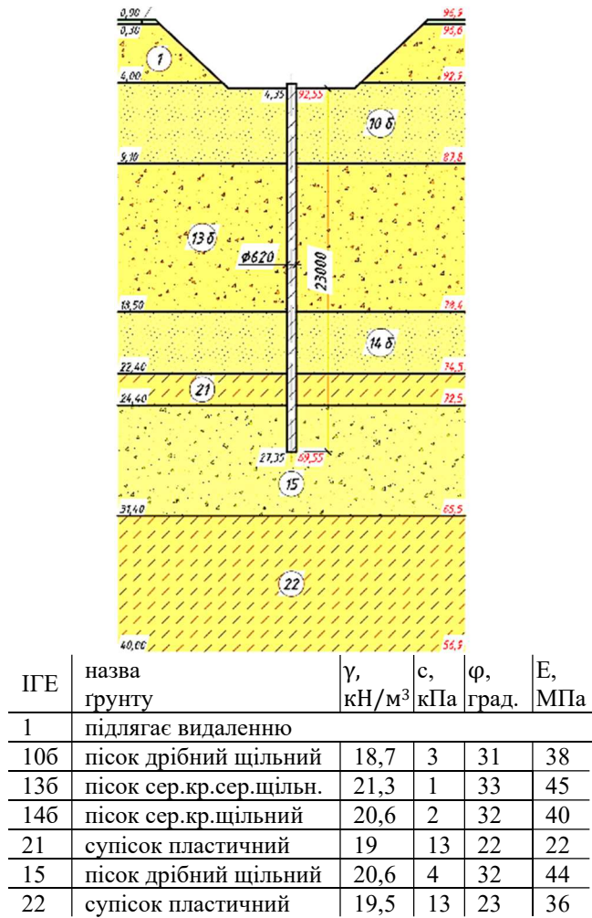
Рис.1. Посадка палі на геологію
