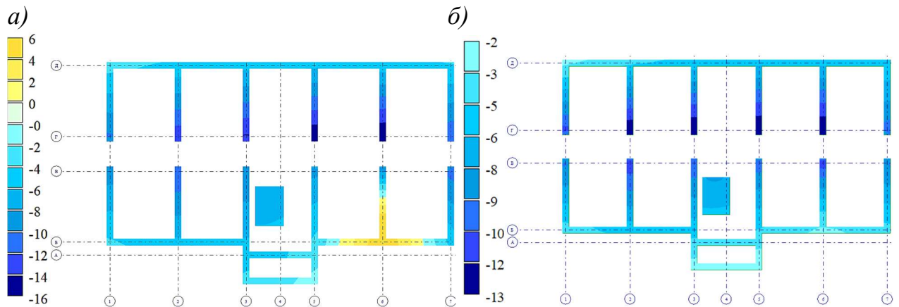
Рис. 11. Осідання ростверків пальових фундаментів для сценарію локальної відмови стінової панелі 1-го поверху (квазістатична постановка), s , мм: а – квазістатична постановка; б – динамічна постановка
