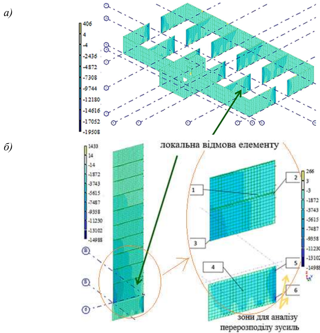
Рис. 9. Поздовжні зусилля N_y в стінах секції будинку для умов нормальної експлуатації, \text{кН/м}^2 : а – в стінах підвального поверху; б – в стінах по осі «б»
