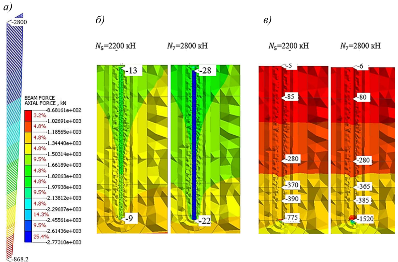
Рис. 4 Результати числового моделювання роботи палі в ґрунті: а – розподіл поздовжнього зусилля в стовбурі палі, N , кН; б - вертикальні переміщення стовбура палі і оточуючого ґрунту, s , мм; в - вертикальні напруження в ґрунті, \sigma_z , кПа
