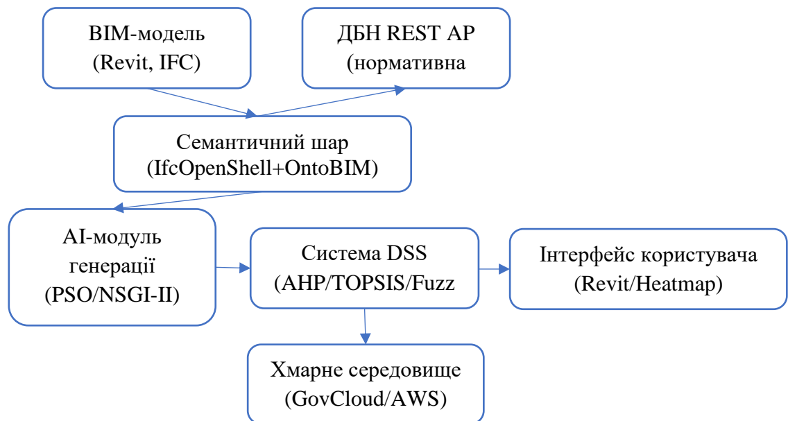
Рисунок 2.4. Архітектурна реалізація системи DSS для AI-BIM Regulatory Intelligence. Джерело: складено автором.
