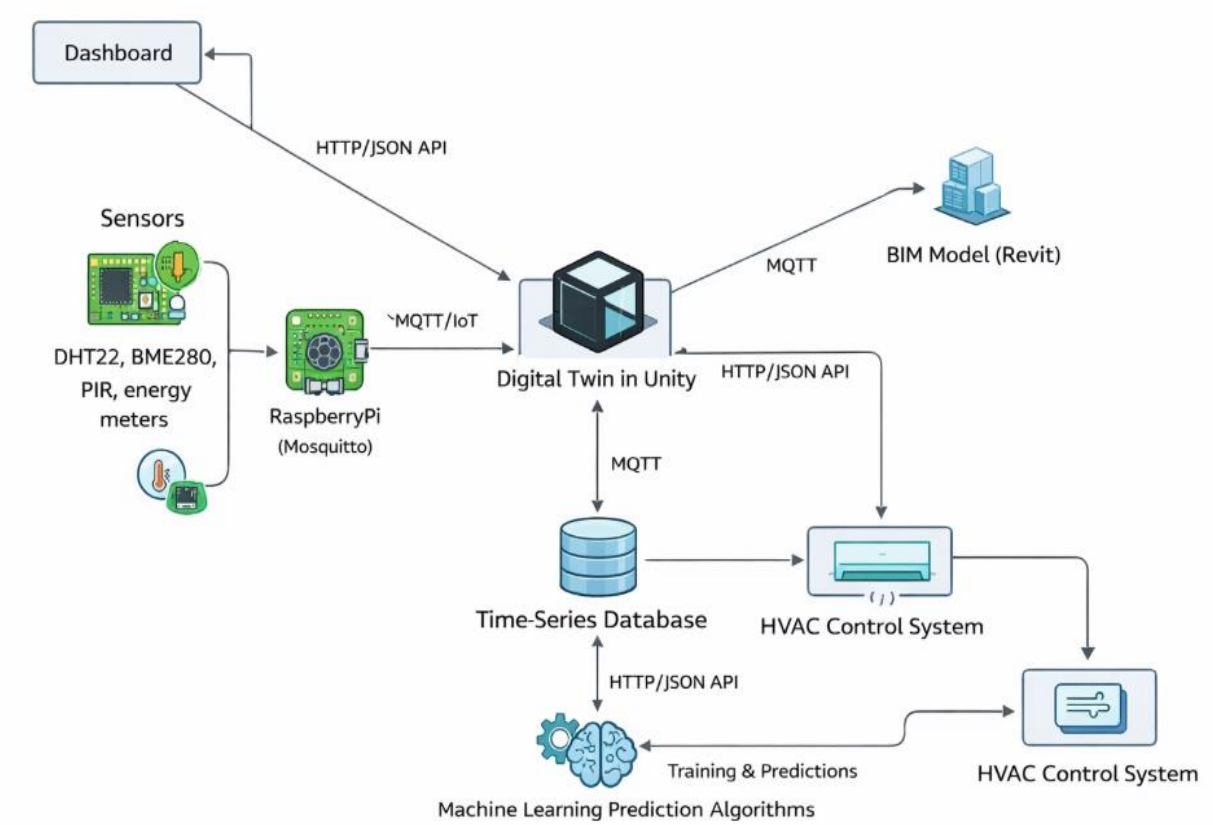
Рисунок Архітектурна схема цифрового двійника будівлі
