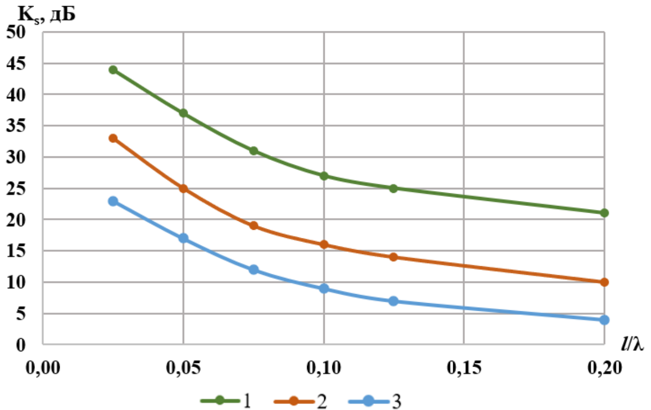
Рис. 3.4 Залежність ефективності екранування сітчастої структури від довжини хвилі екранованого електромагнітного випромінювання, діаметру дроту d та розміру комірки; 1, 2, 3 відповідають співвідношенням l/d=2; 5; 10 , l – відстань між осями дротів
