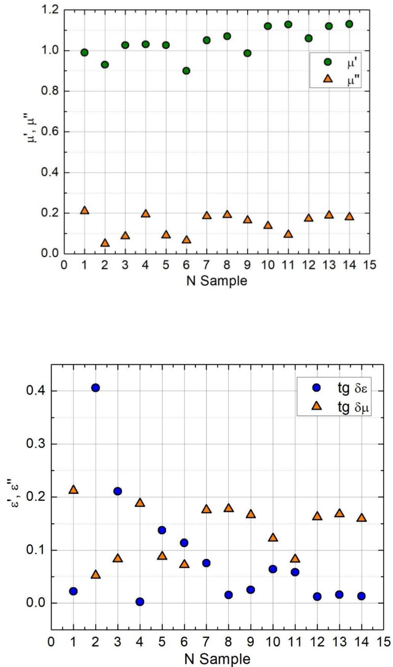
Рис. 3.12. Значення діелектричних і магнітних властивостей композиційних матеріалів за різного вмісту провідних та магнітних компонентів.
