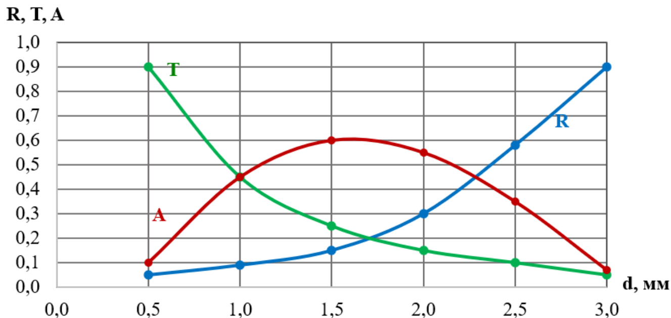
Рис. 3.15 Співвідношення коефіцієнтів проходження T та відбиття R у залежності від товщини захисного шару ( f = 2,45 ГГц)
