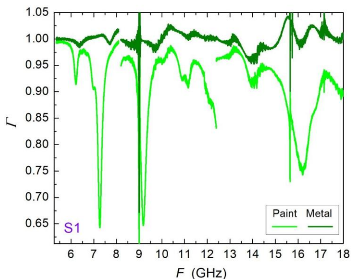
Рис. 3.10. Залежність коефіцієнта відбиття від частоти екранованого електромагнітного випромінювання, — – підкладка, — – покриття
