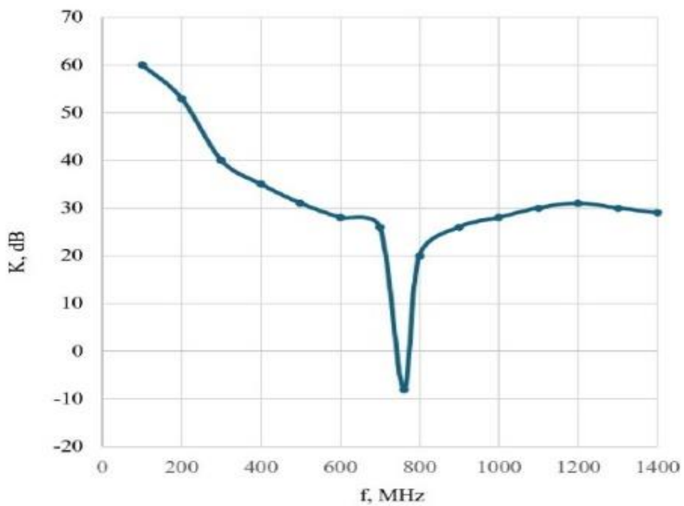
Рис. 3.8. Результати випробувань конструкції з отвором розмірами 20 \times 3 см.
