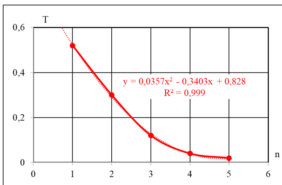
Рис. 3.2. Залежність коефіцієнта пропускання регулярної структури ( T ) від кількості шарів ( n ), частота електромагнітного випромінювання 3 ГГц
