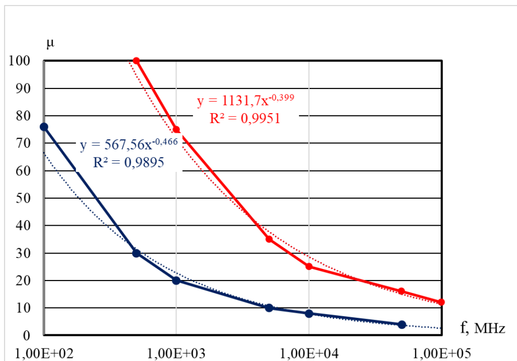
Рис. 3.3. Частотні залежності магнітної проникності за поглинанням \mu_k та за заломленням \mu_n конструкційної сталі марки 45: —●— — магнітної проникності за поглинанням \mu_k ; —●— — магнітної проникності за заломленням \mu_n
