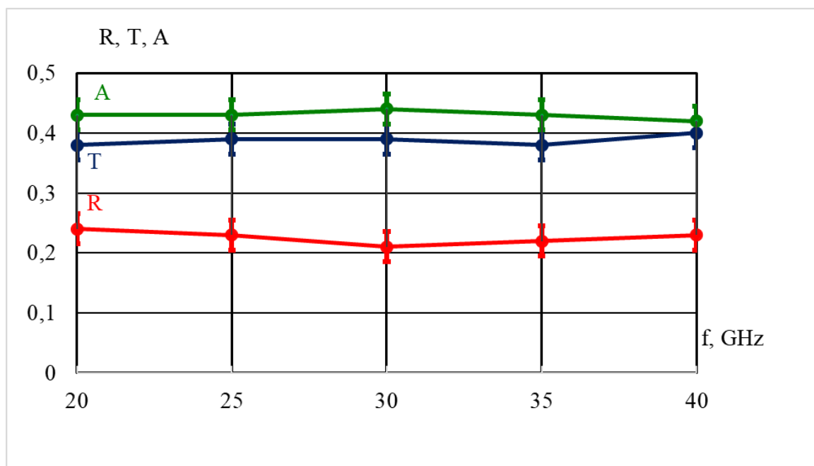
Рис. 3.13. Коефіцієнти відбиття ( R ), проходження ( T ) та поглинання ( A ) одношарового матеріалу завтовшки 5 мм з вмістом карбонільного заліза 14–15 % за об'ємом
