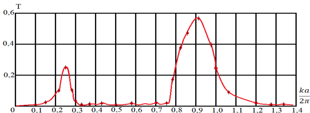
Рис. 3.1. Амплітудно-частотна залежність коефіцієнта пропускання електромагнітної хвилі ( T ) конструкції з одним рядом металевих стрижнів
