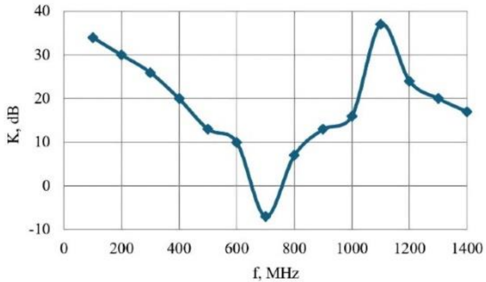
Рис. 3.7. Залежність коефіцієнта екранування металевої конструкції з отвором розміром 10 \times 1 см від частоти екранованого електромагнітного поля.
