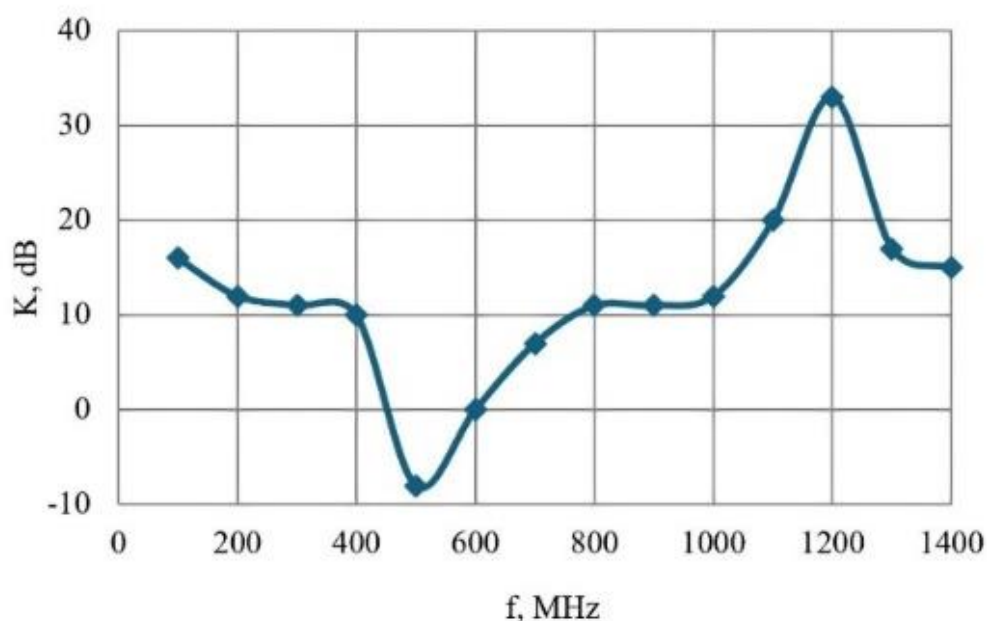
Рис 3.6. Залежність коефіцієнта екранування металеві конструкції з отвором розміром 15 \times 5 см від частоти екранованого електромагнітного поля.
