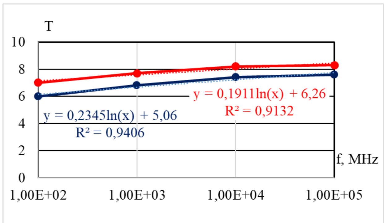
Рис. 3.9. Частотна залежність коефіцієнтів пропускання ( T ) електромагнітного випромінювання діелектричними матеріалами: —●— суцільний цементобетон; —●— сітчаста базальтова структура у цементобетонній матриці
