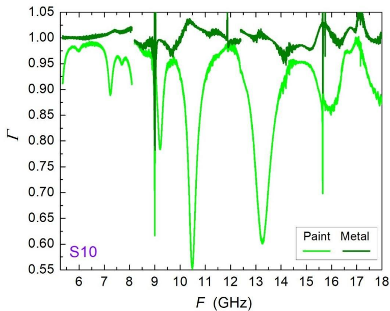
Рис. 3.11. Частотна залежність коефіцієнта відбиття тонких композиційних матеріалів різних складів
